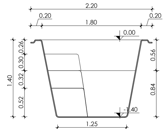
Corte Transversal Esc.: 1:40
