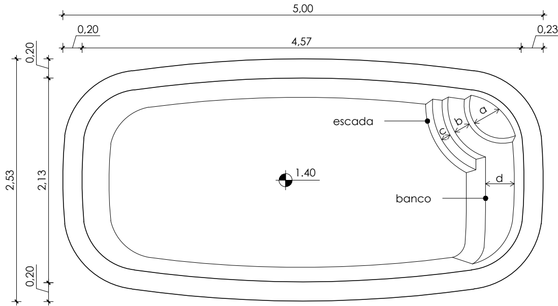
Planta Baixa Esc.: 1:40
