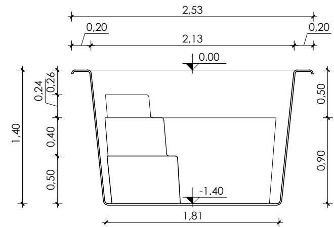
Corte Transversal Esc.: 1:40
