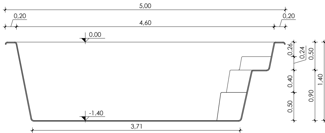
Corte Longitudinal Esc.: 1:40
