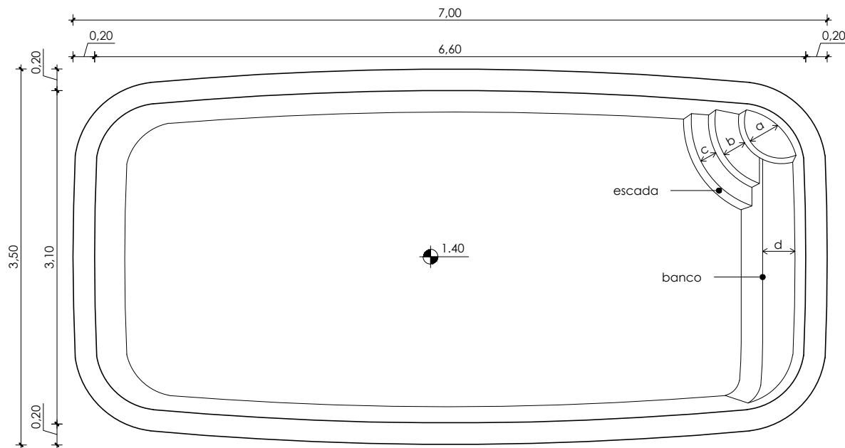
Planta Baixa Esc.: 1:50
