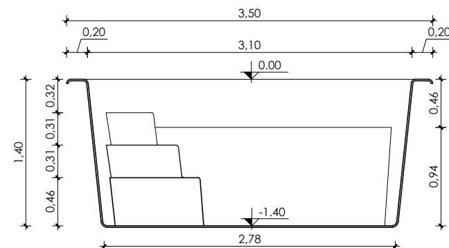
Corte Transversal Esc.: 1:50
