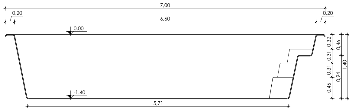
Corte Longitudinal Esc.: 1:50
