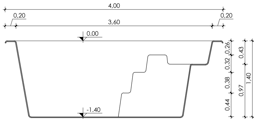
Corte Longitudinal Esc.: 1:40
