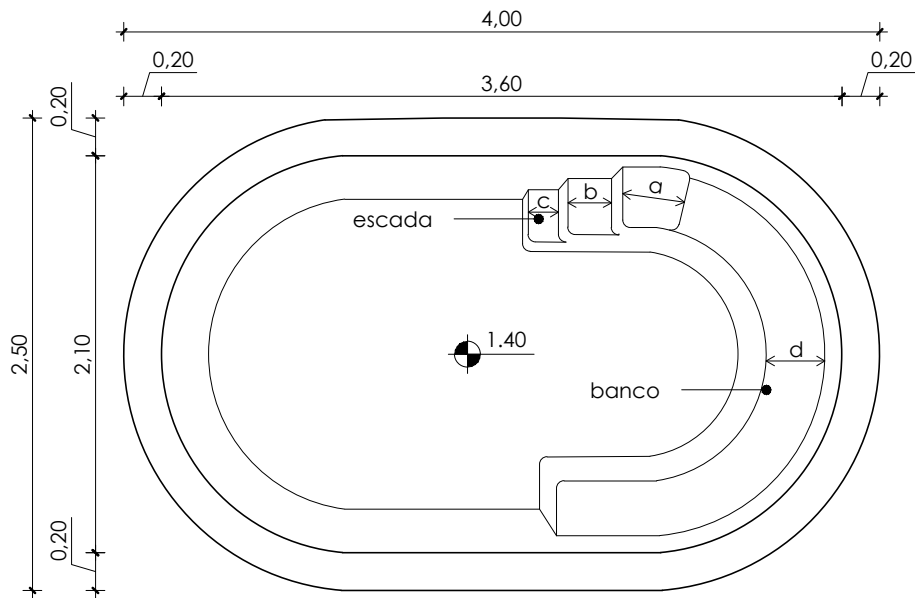
Planta Baixa Esc.: 1:40
