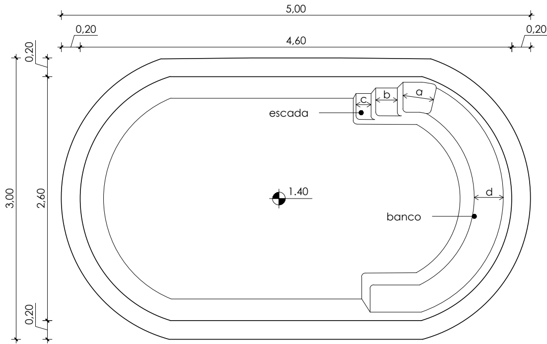
Planta Baixa Esc.: 1:40
