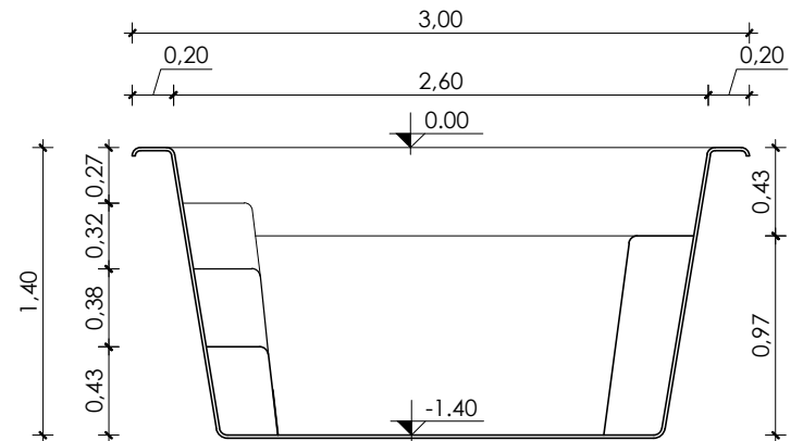
Corte Transversal Esc.: 1:40
