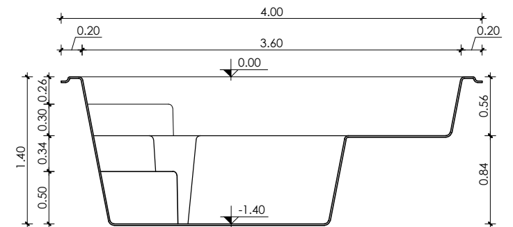
Corte Transversal Esc.: 1:50
