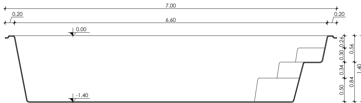
Corte Longitudinal Esc.: 1:50
