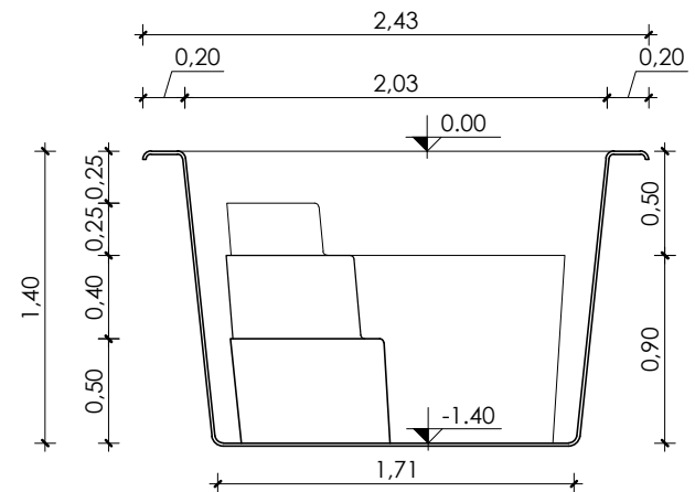
Corte Transversal Esc.: 1:40
