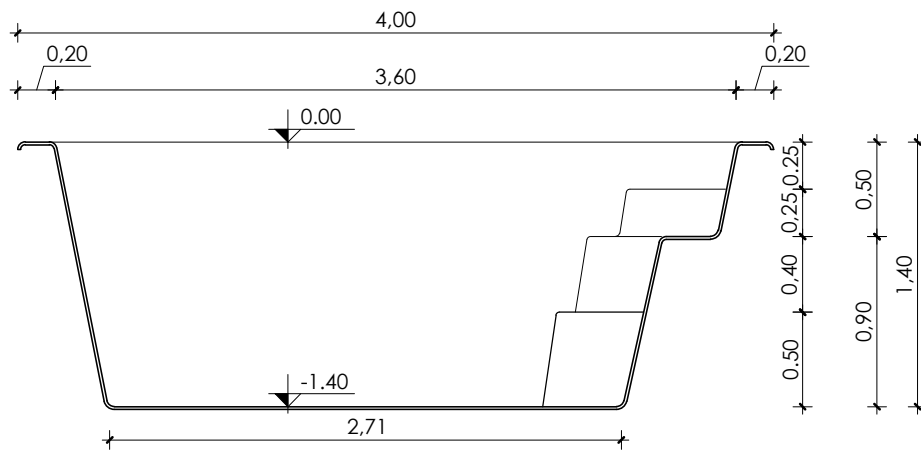
Corte Longitudinal Esc.: 1:40
