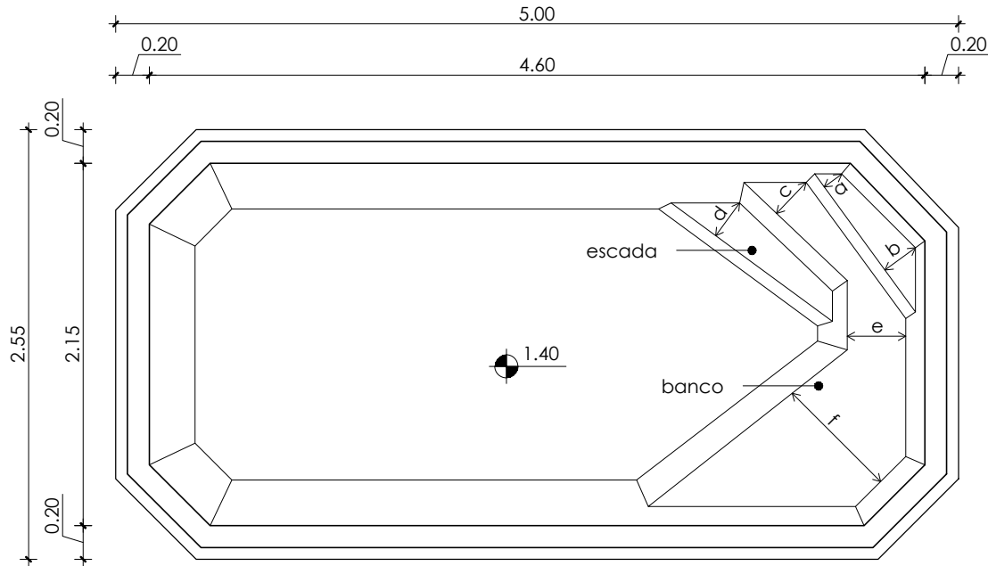
Planta Baixa Esc.: 1:40
