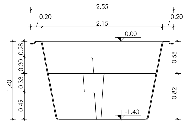
Corte Transversal Esc.: 1:40
