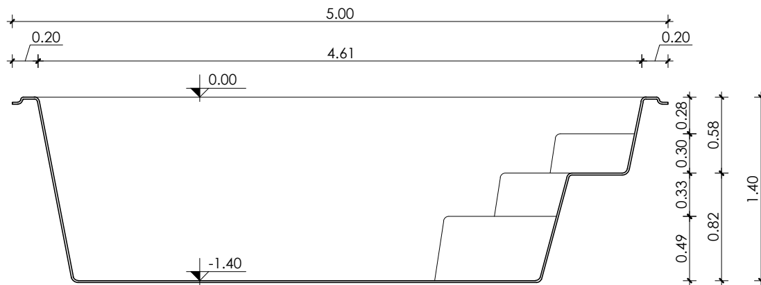
Corte Longitudinal Esc.: 1:40
