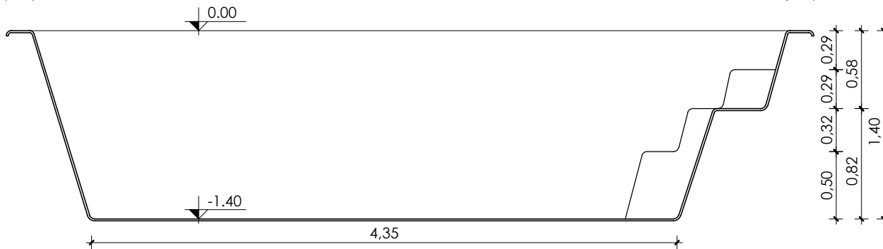
Corte Longitudinal Esc.: 1:40
