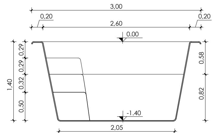
Corte Transversal Esc.: 1:40
