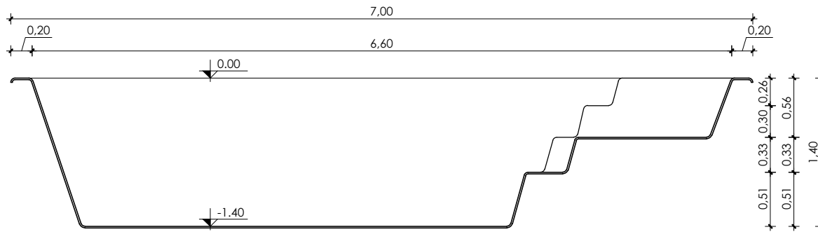
Corte Longitudinal Esc.: 1:50
