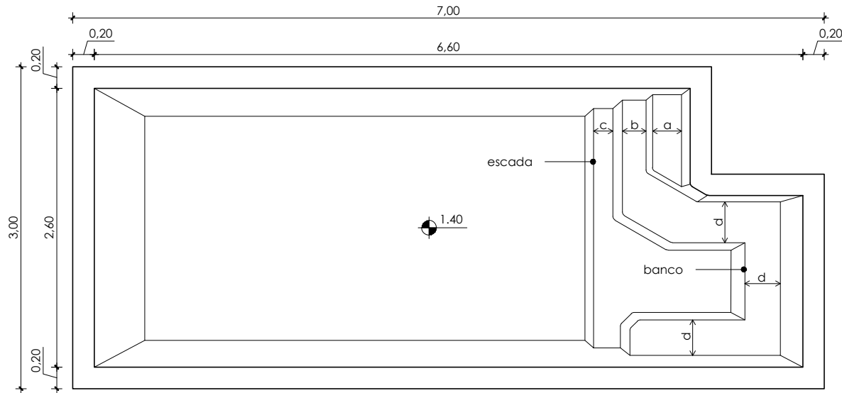
Planta Baixa Esc.: 1:50
