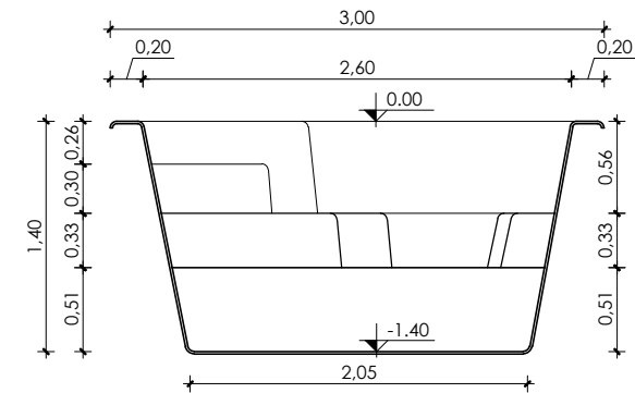
Corte Transversal Esc.: 1:50
