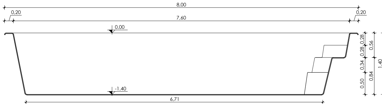
Corte Longitudinal Esc.: 1:50
