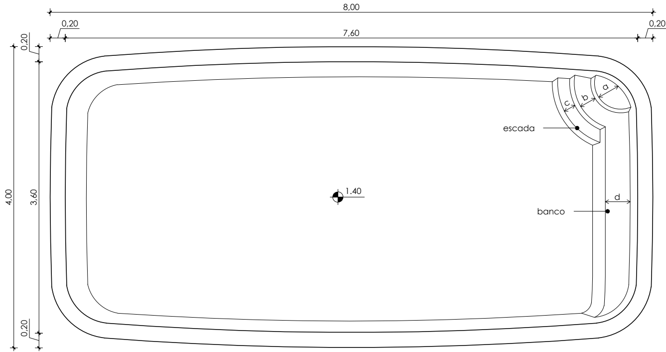
Planta Baixa Esc.: 1:50
