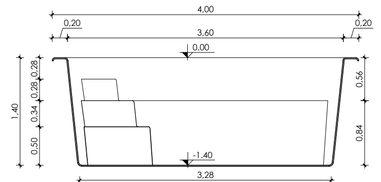
Corte Transversal Esc.: 1:50
