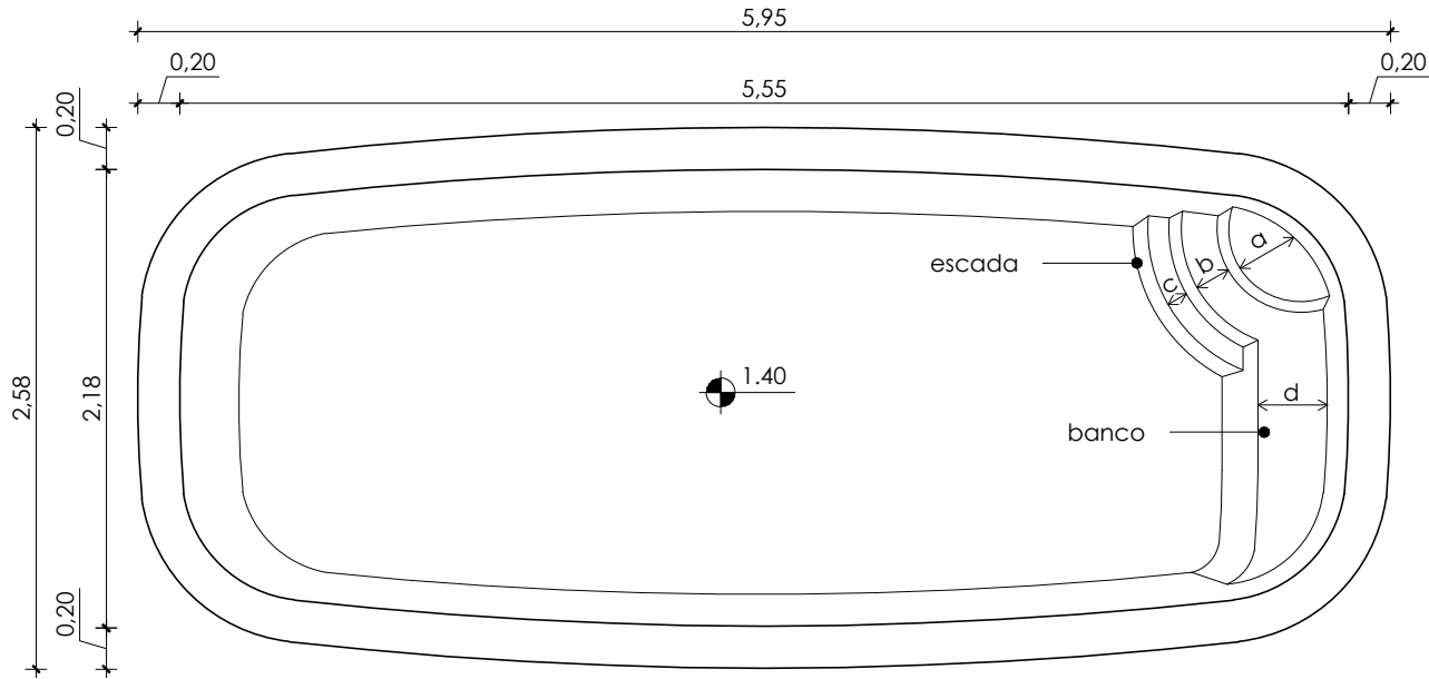
Planta Baixa Esc.: 1:40
