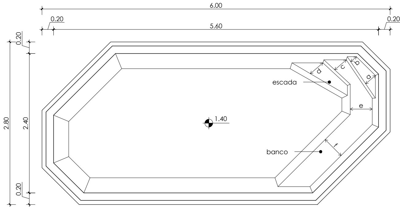
Planta Baixa Esc.: 1:40
