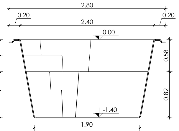
Corte Transversal Esc.: 1:40
