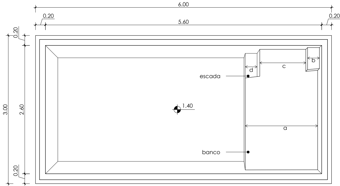
Planta Baixa Esc.: 1:40
